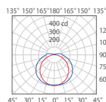
LB5D-△△H65E 6500K
