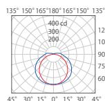
LB5D-△△H50E 5000K
