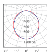
FB25J-50H 5000K 3380 lm
