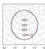
FB25J-65H 6500K 3380 lm
